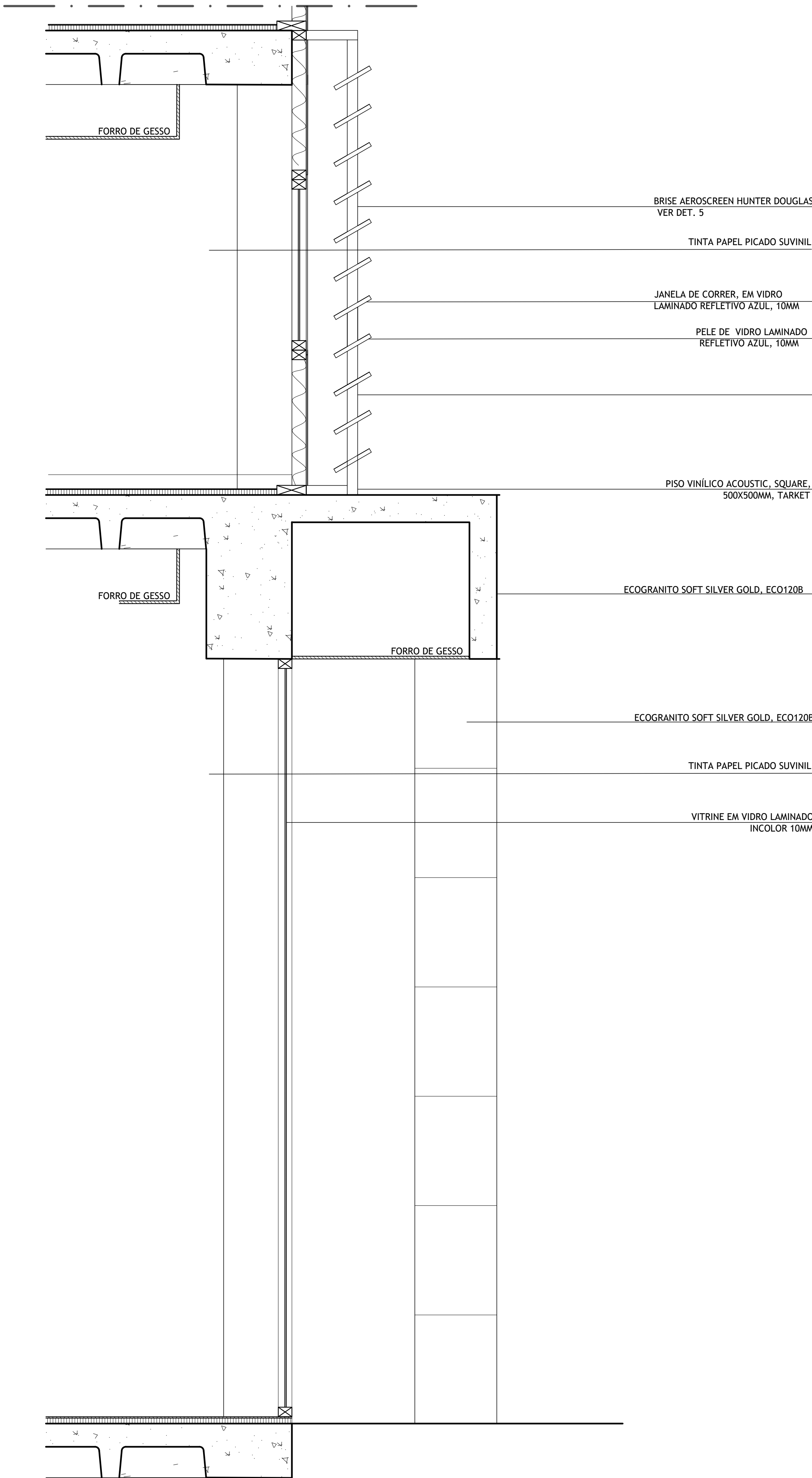
CORTE DD - SEÇÃO B ESCALA 1/20
