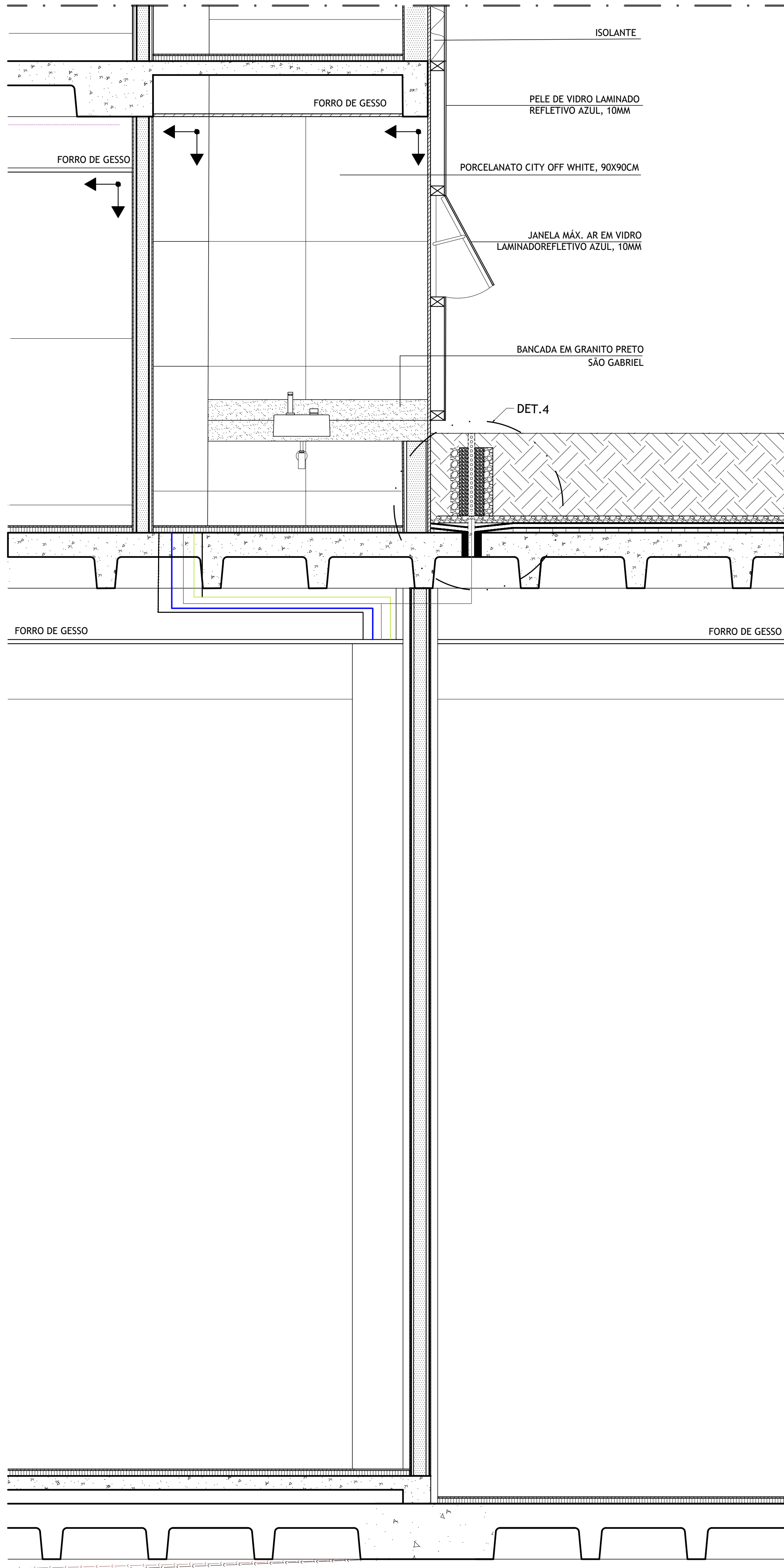
CORTE AA - SEÇÃO B ESCALA 1/20
