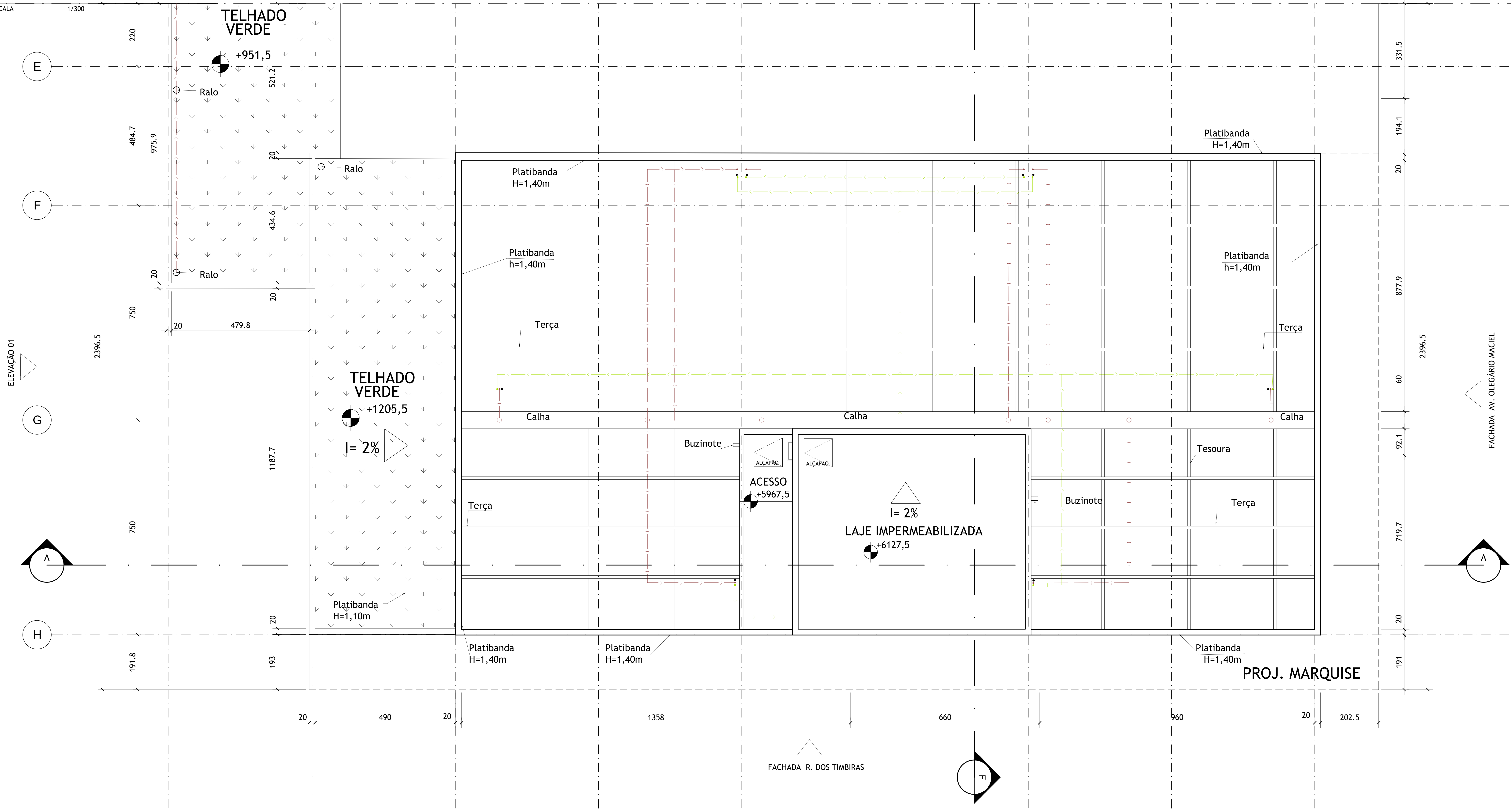
PLANTA CHAVE - ENGRADAMENTO ESCALA 1/300
