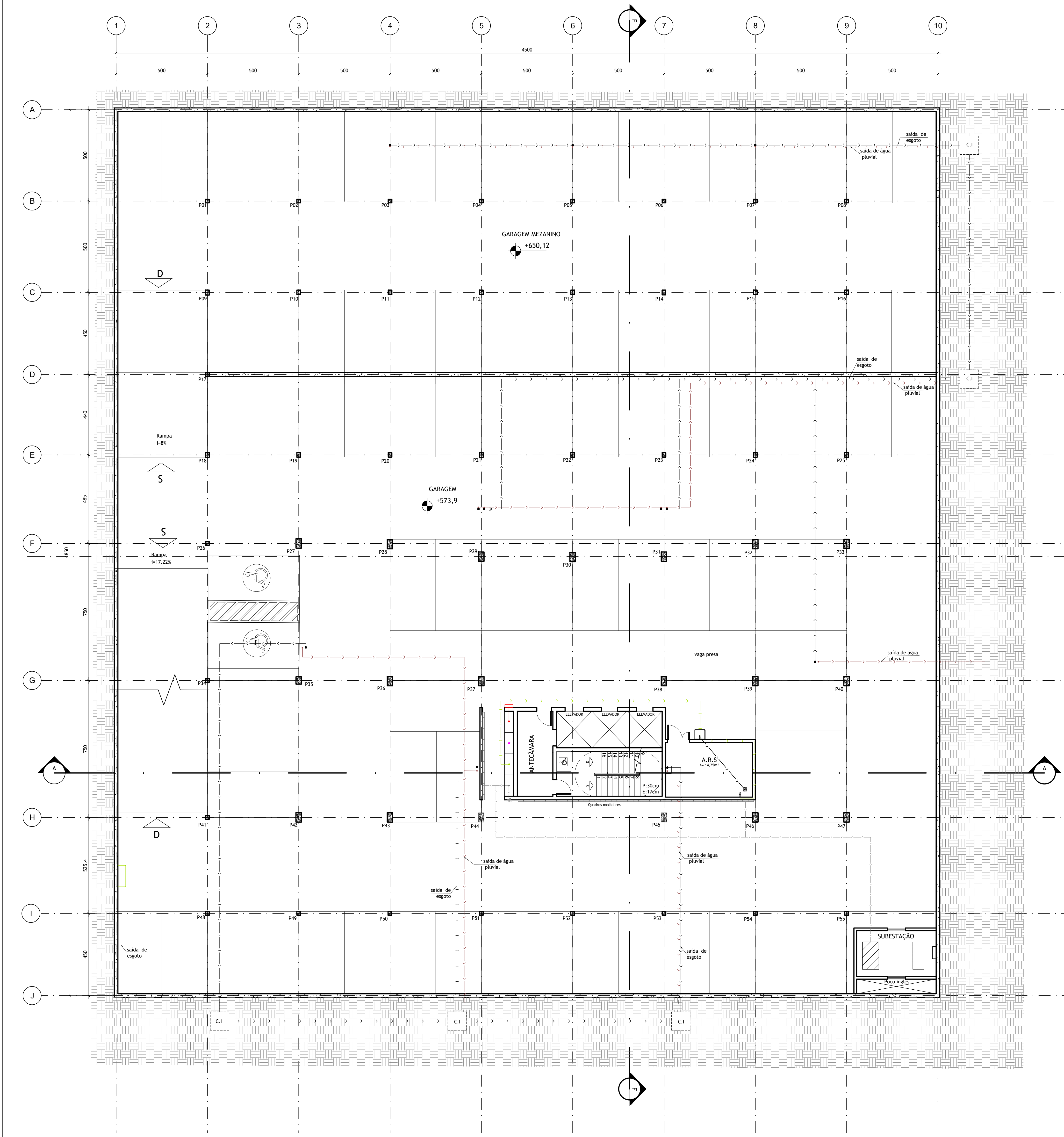
PLANTA GARAGEM 1 PAVIMENTO ESCALA: 1/100
