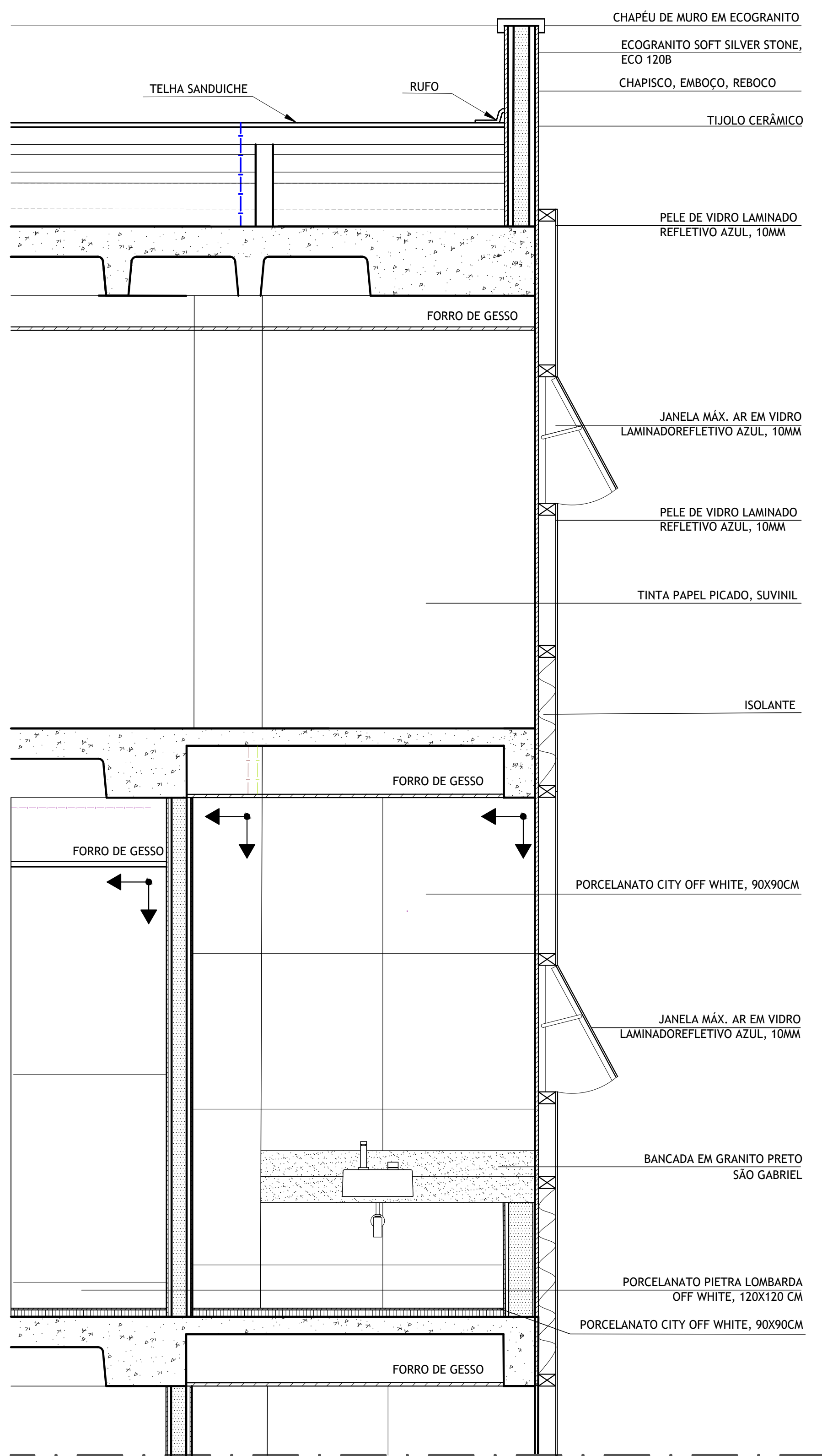
CORTE AA - SEÇÃO A ESCALA 1/20
