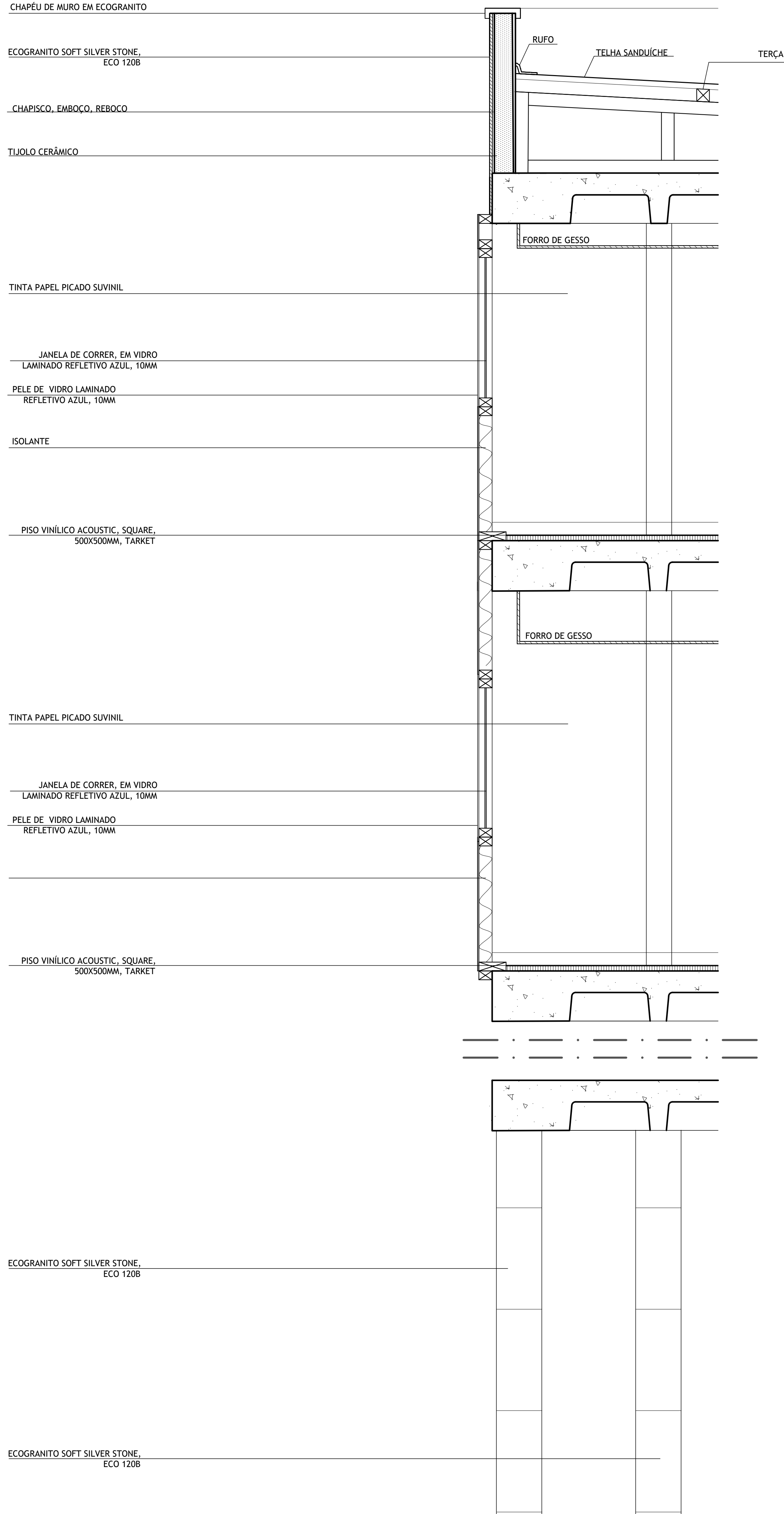
CORTE BB - SEÇÃO A ESCALA 1/20
