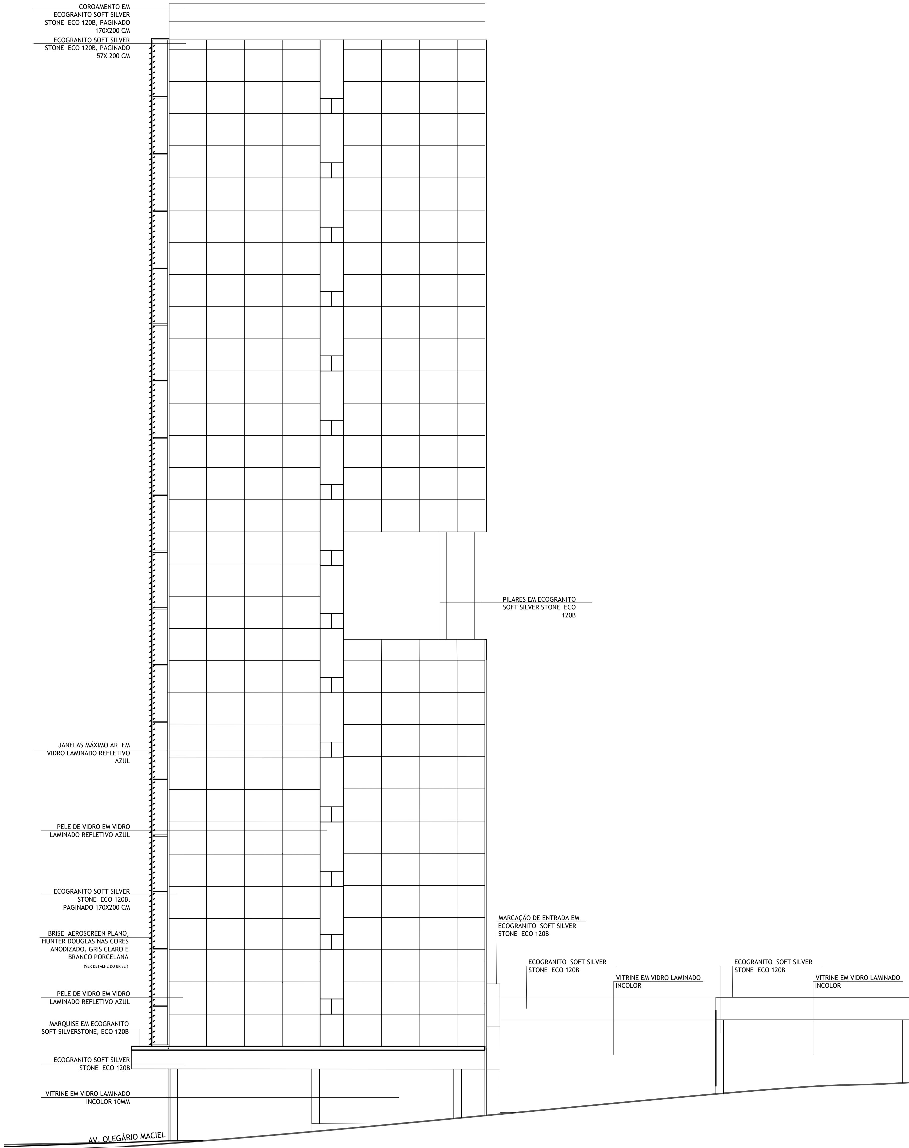
FACHADA 1- AV. OLEGÁRIO MACIEL ESCALA: 1/100
