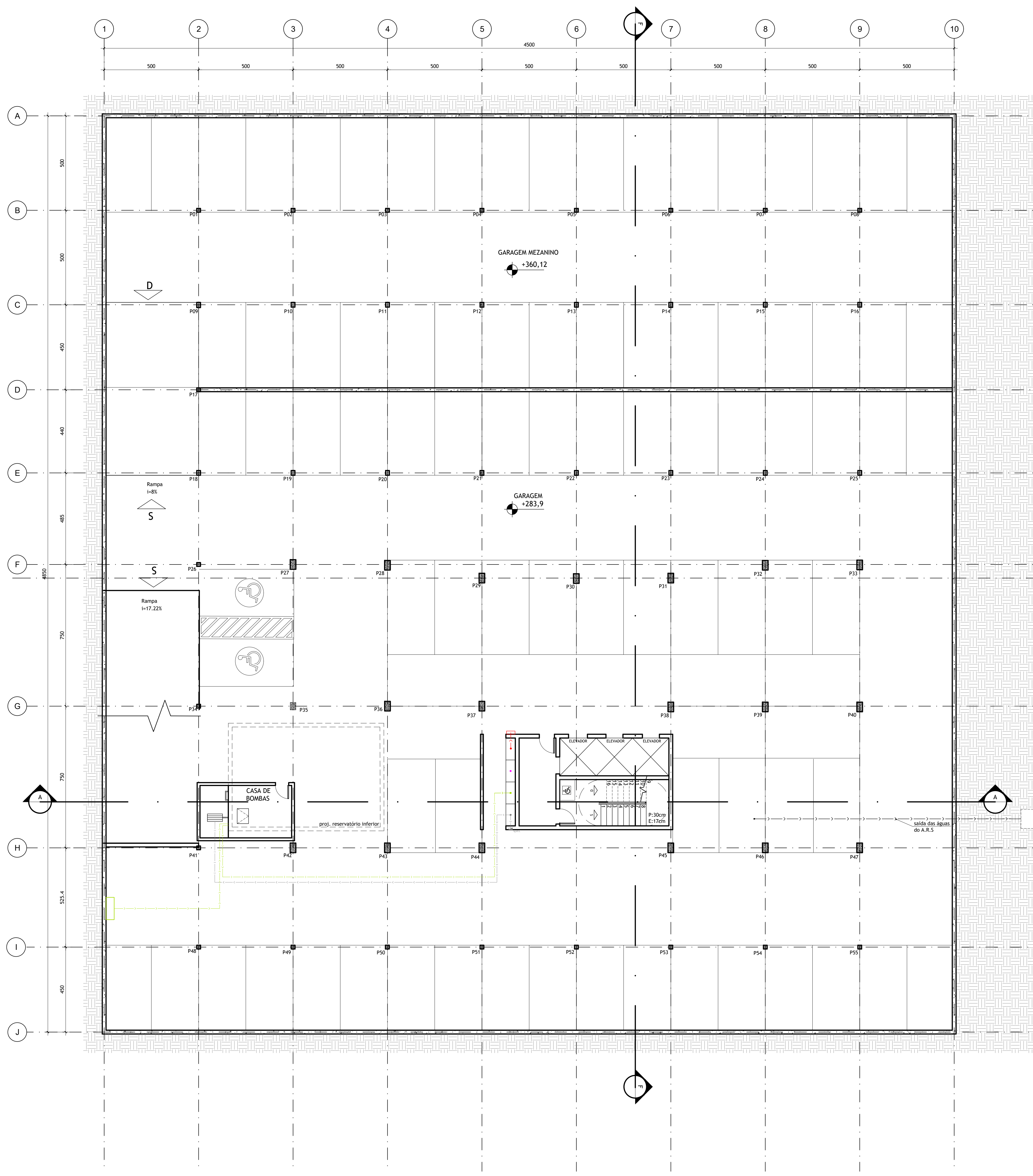
PLANTA GARAGEM 2 PAVIMENTO ESCALA: 1/100
