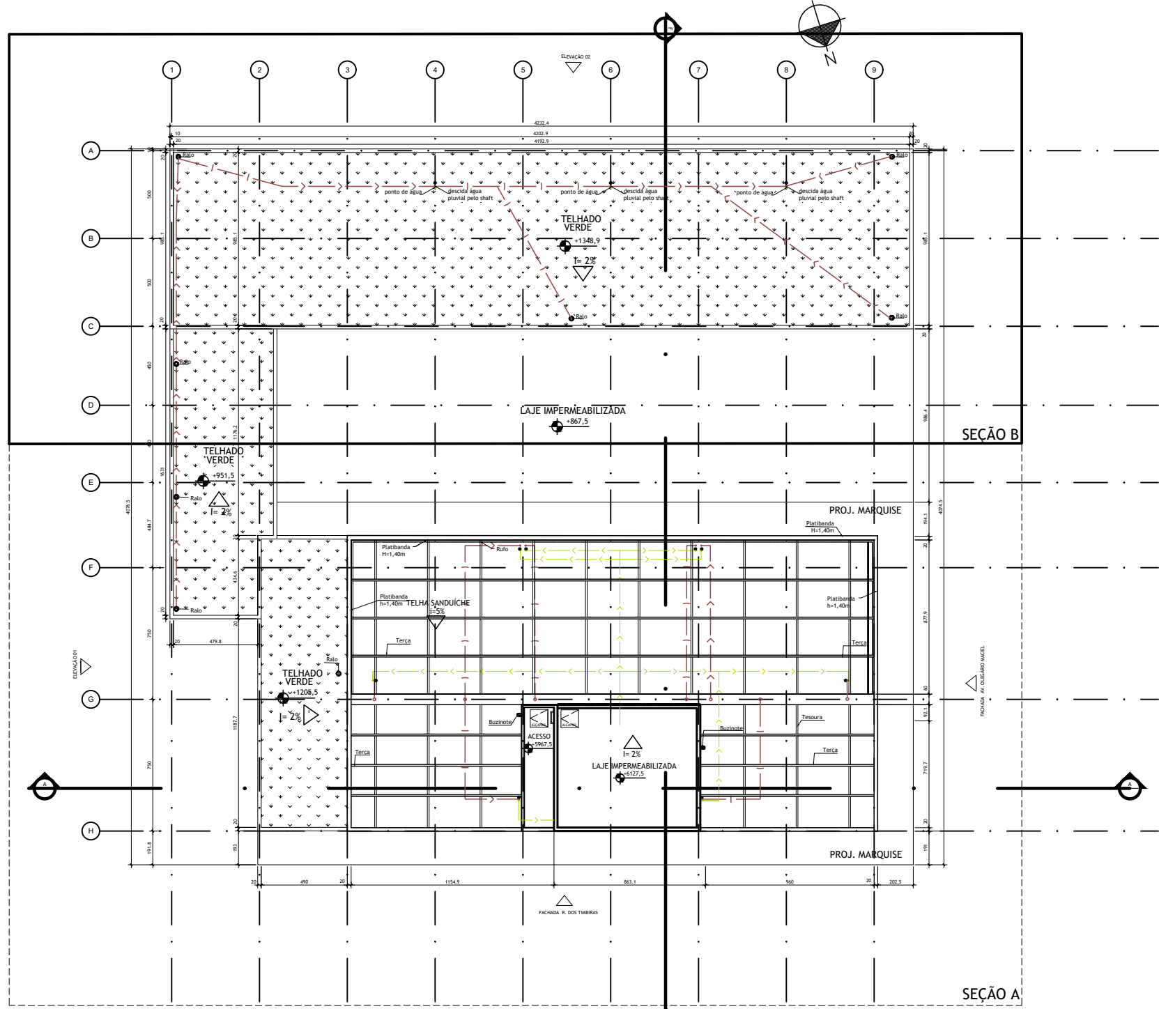
PLANTA CHAVE - ENGRADAMENTO ESCALA 1/300
