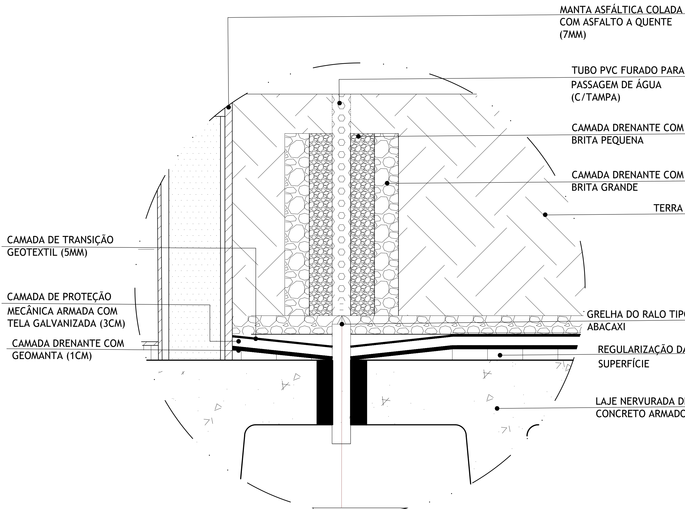
DET 04. TELHADO VERDE ESCALA: 1/5
