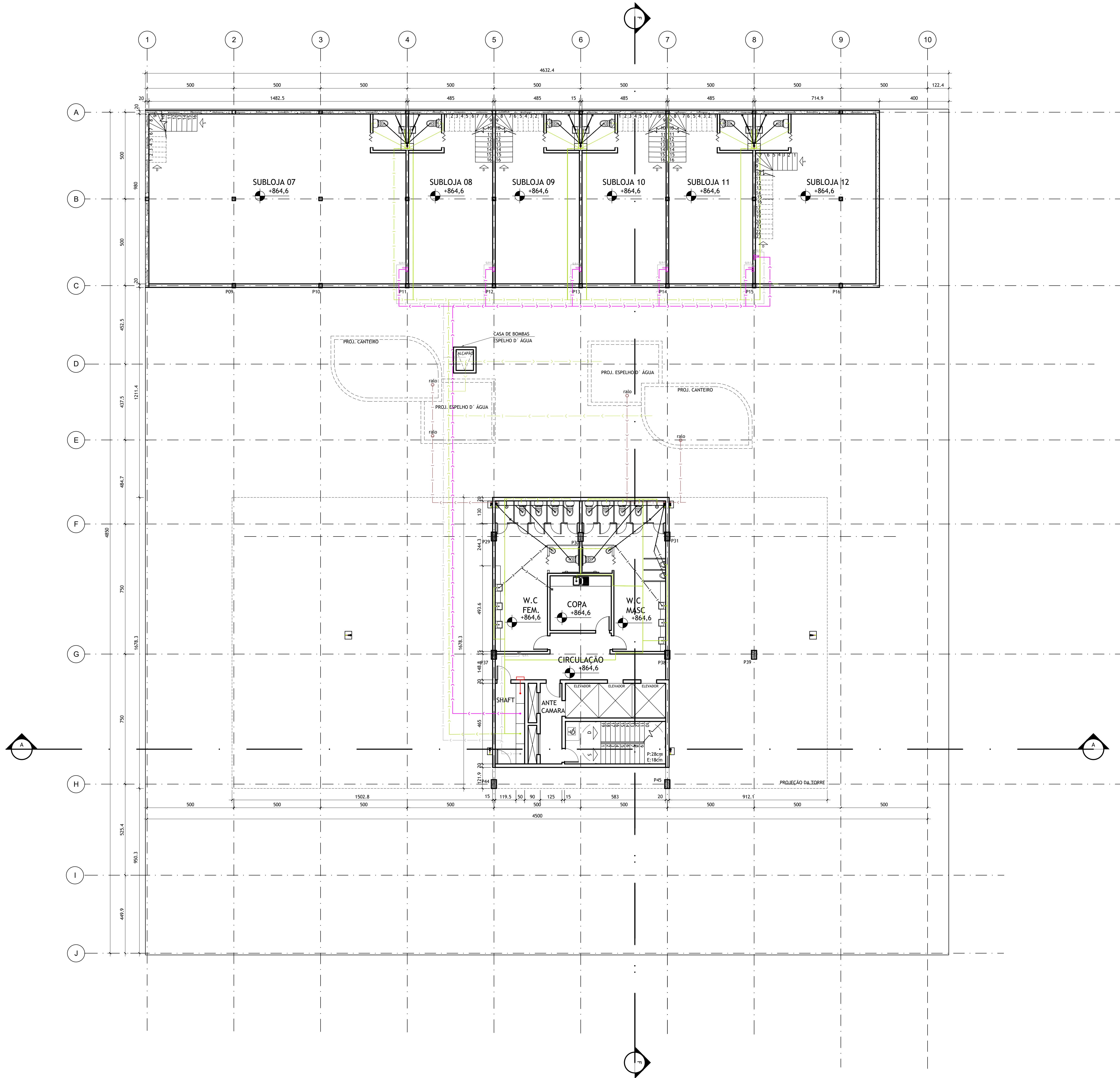
PLANTA LOJAS, W.C E COPA ESCALA: 1/100
