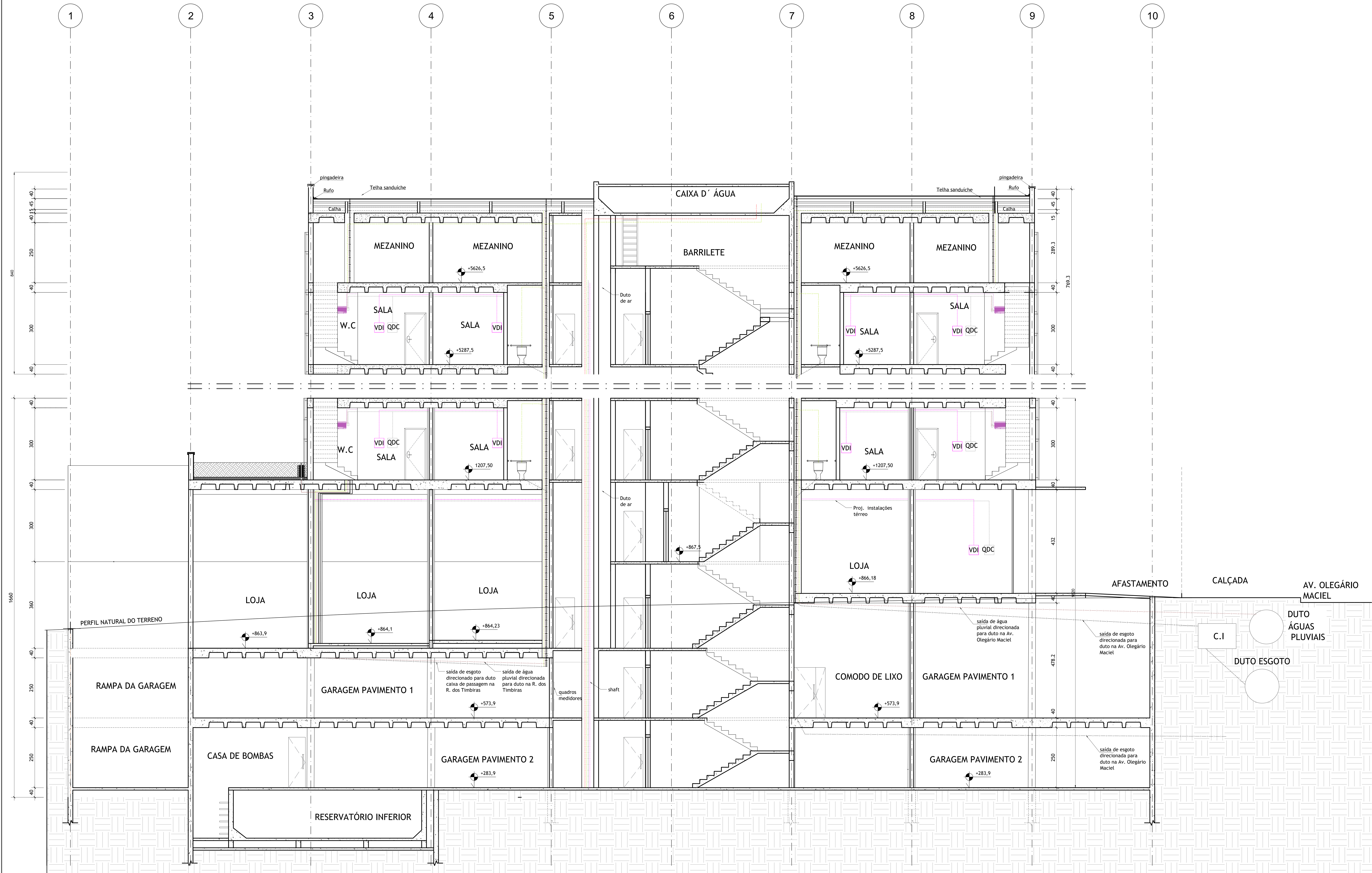
CORTE AA- TRANSVERSAL
