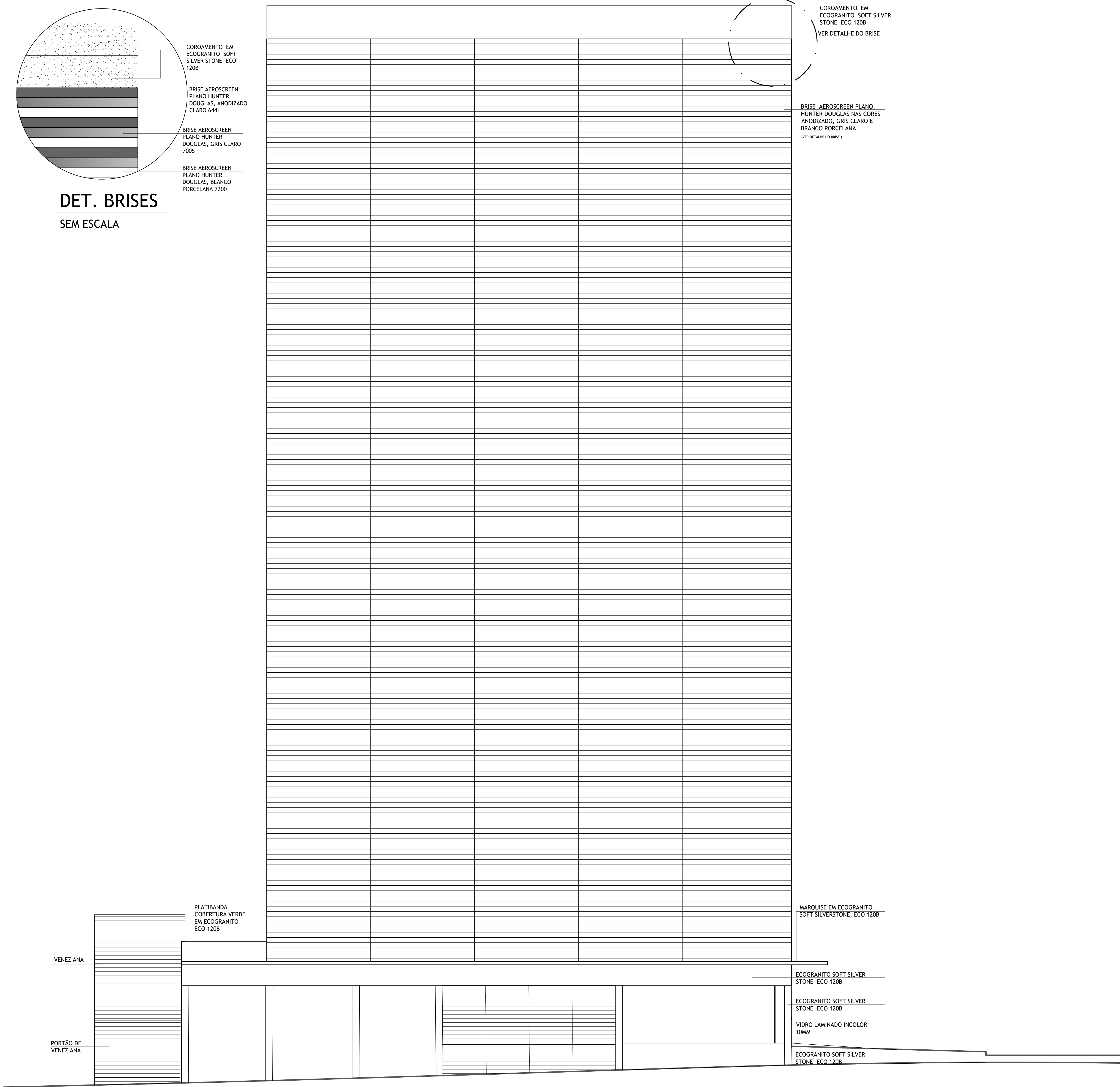
FACHADA 2- RUA DOS TIMBIRAS ESCALA: 1/100
