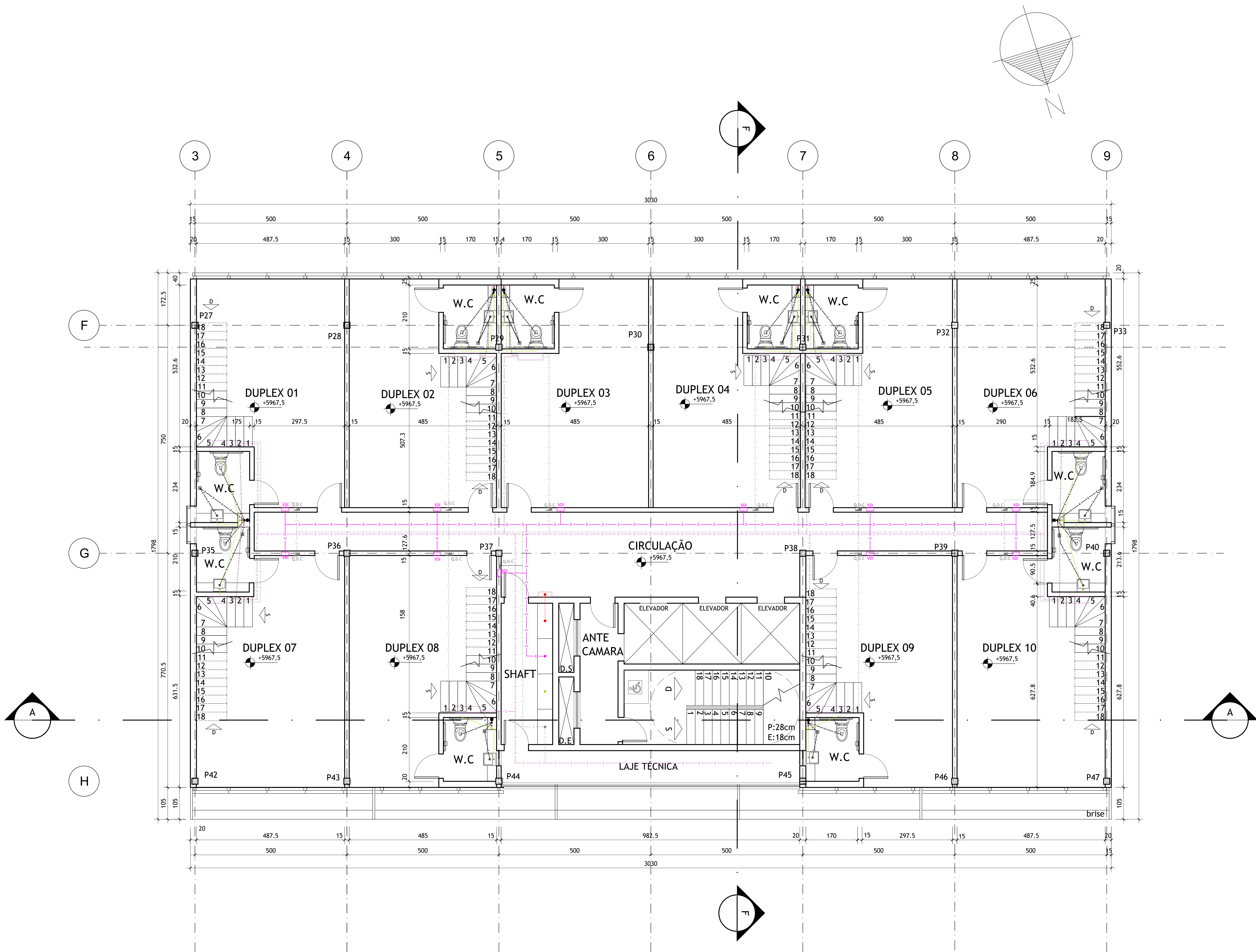
PLANTA SALAS DUPLEX ESCALA: 1/50
