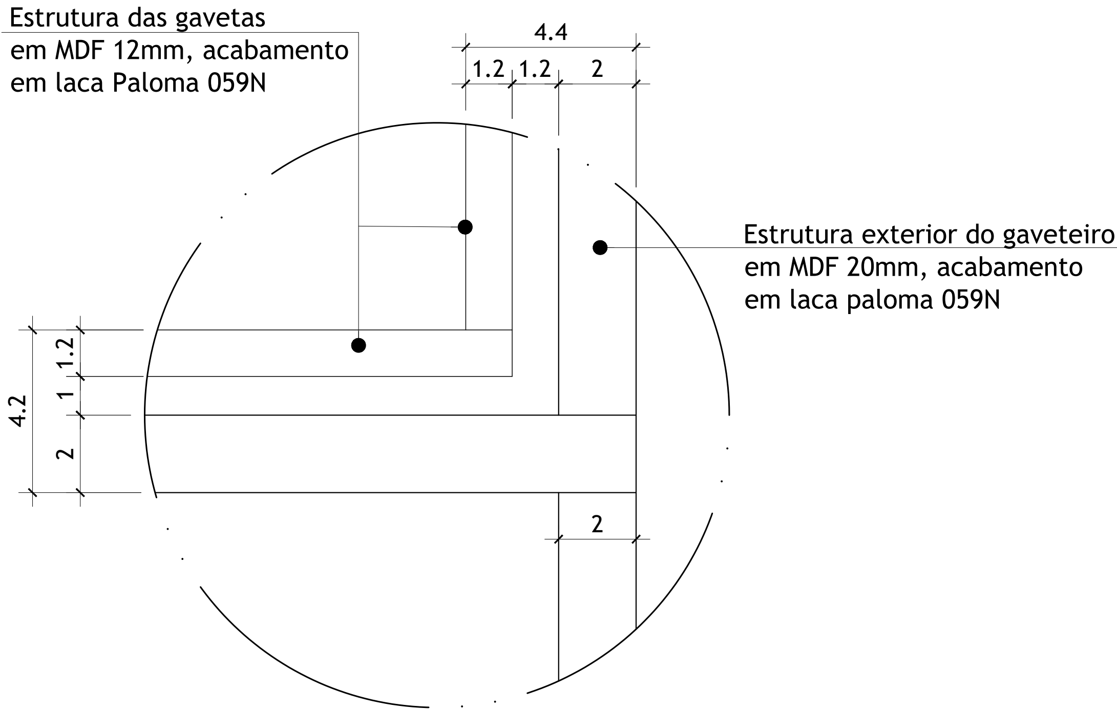
DET 07- GAVETEIRO ESCALA 1:1
