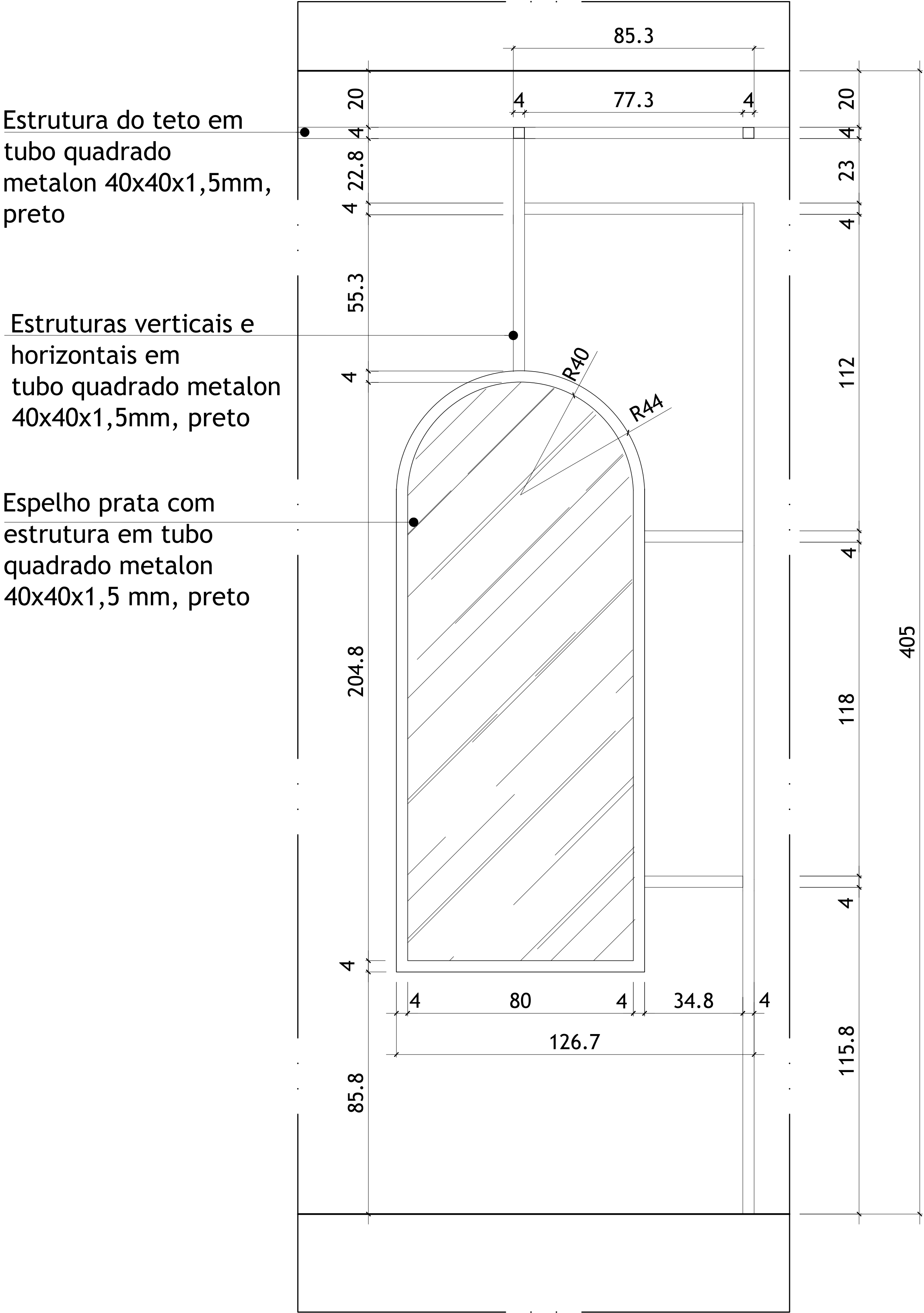
VISTA FRONTAL ESPELHO ESCALA 1:10
