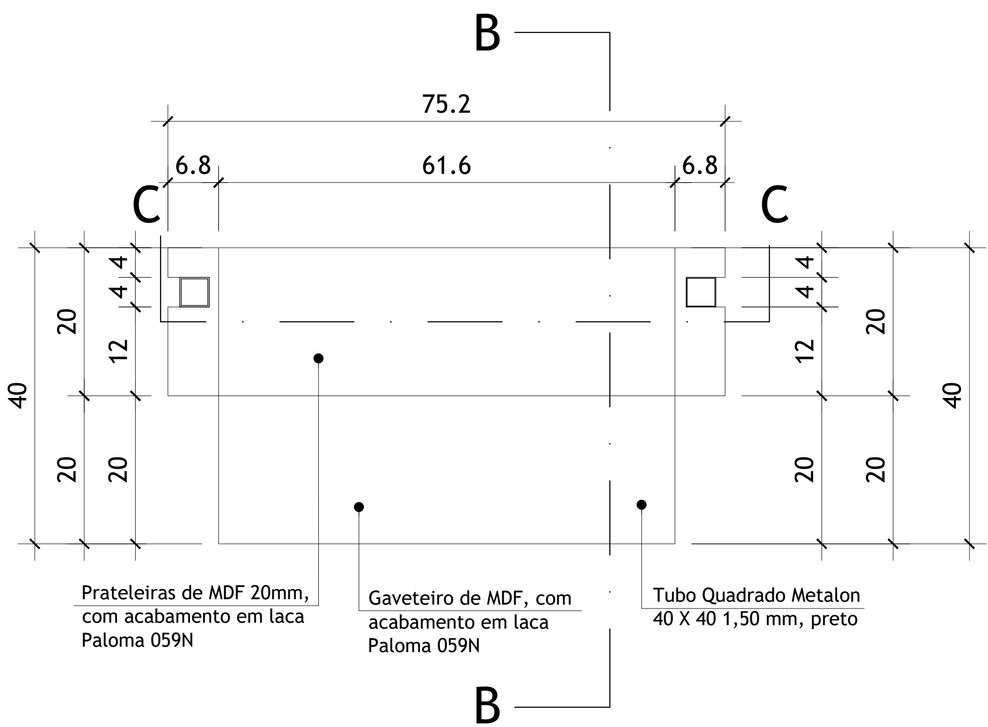
PLANTA DO GAVETEIRO ESCALA 1:5
