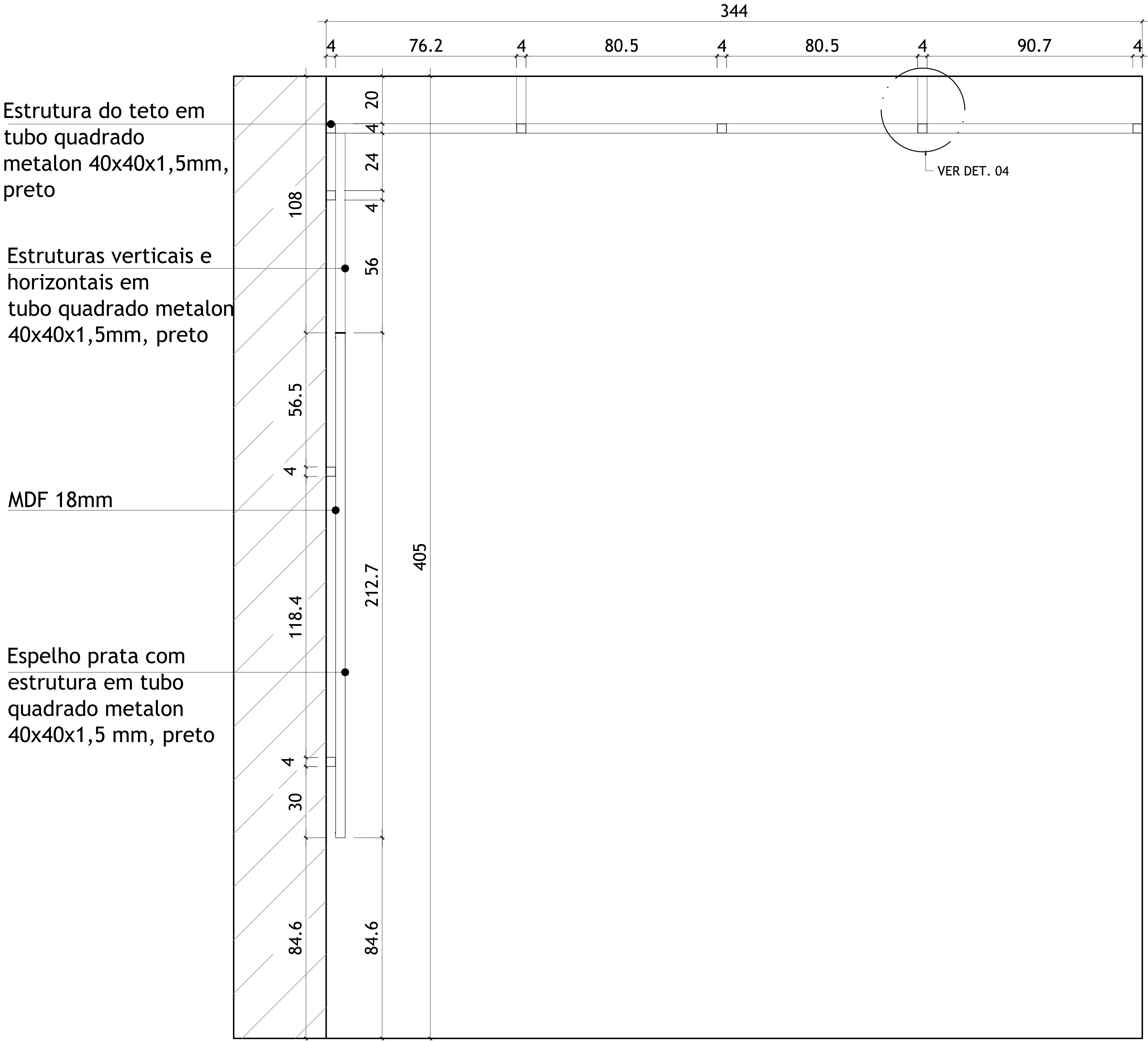
VISTA LATERAL ESPELHO ESCALA 1:10
