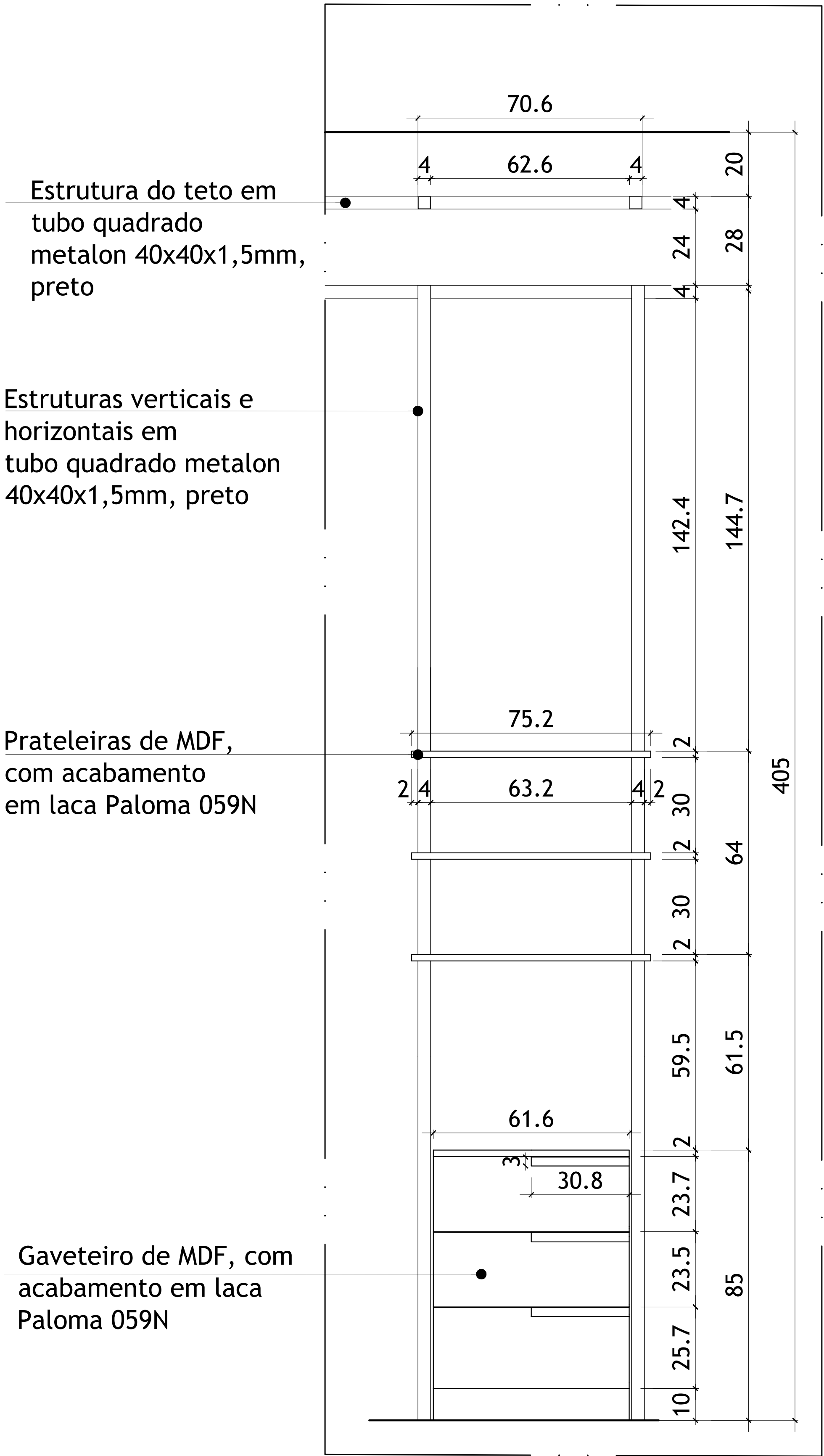
VISTA FRONTAL GAVETEIRO ESCALA 1:10
