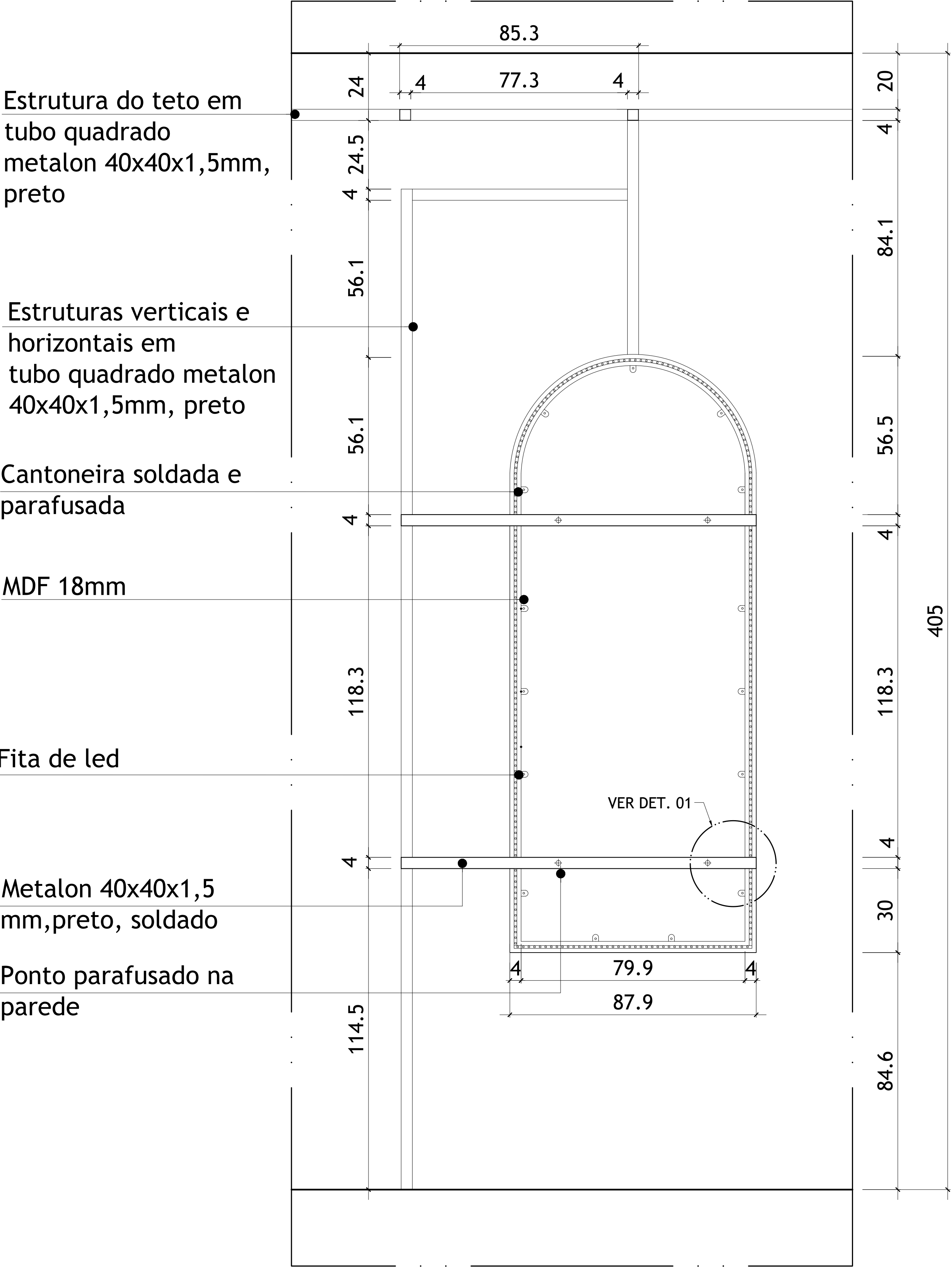
VISTA POSTERIOR ESPELHO ESCALA 1:10
