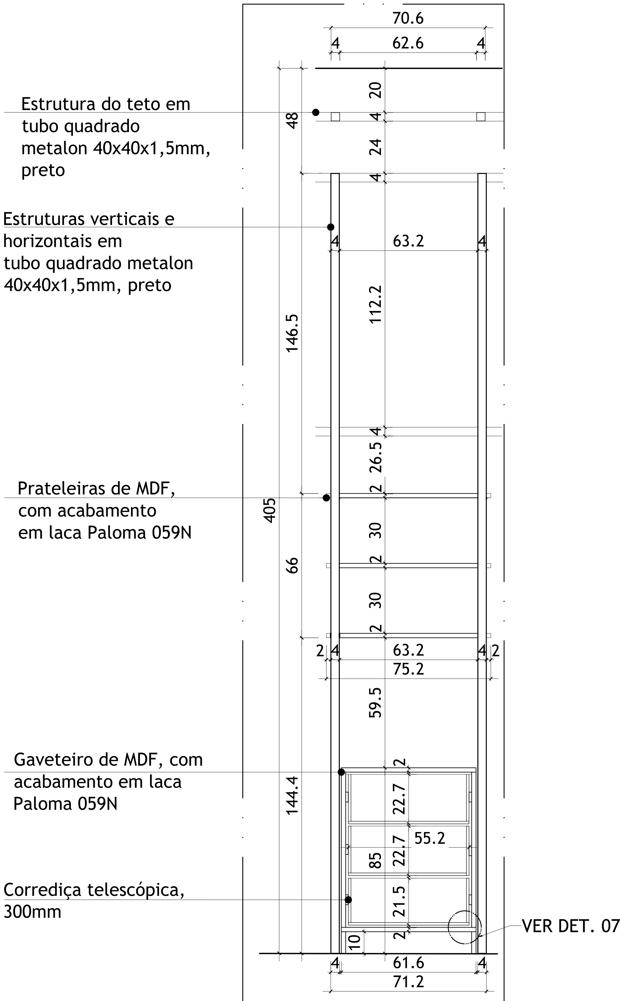
CORTE CC ESCALA 1:10
