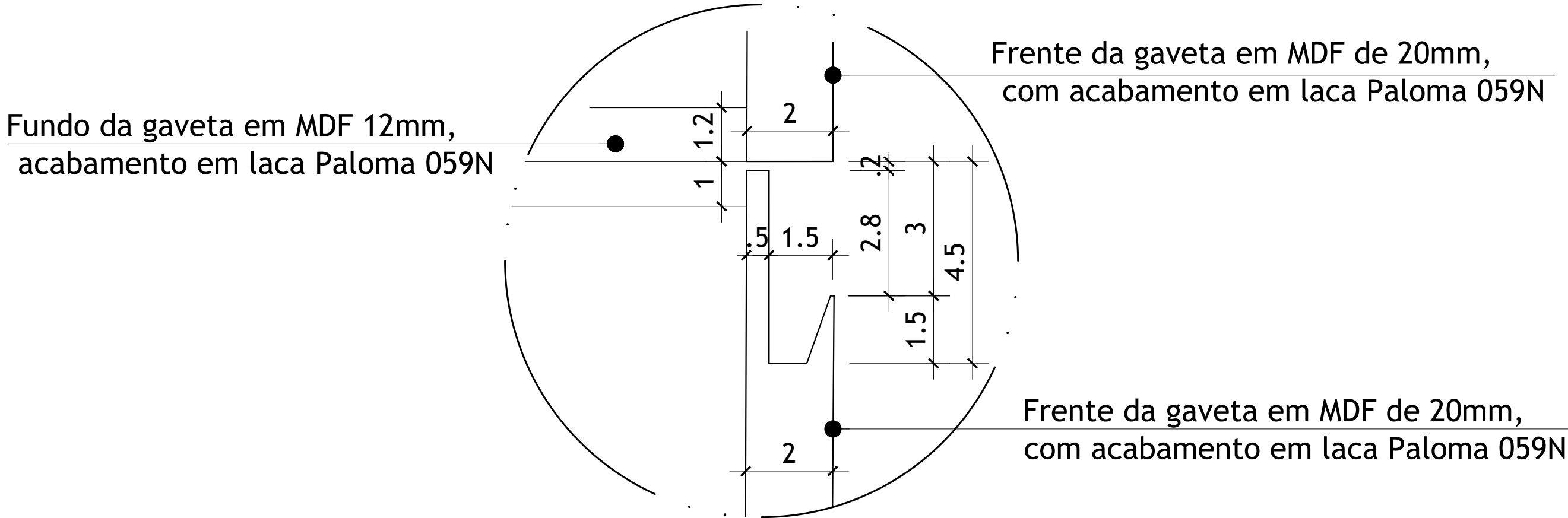
DET 05- PUXADOR CAVA ESCALA 1:1
