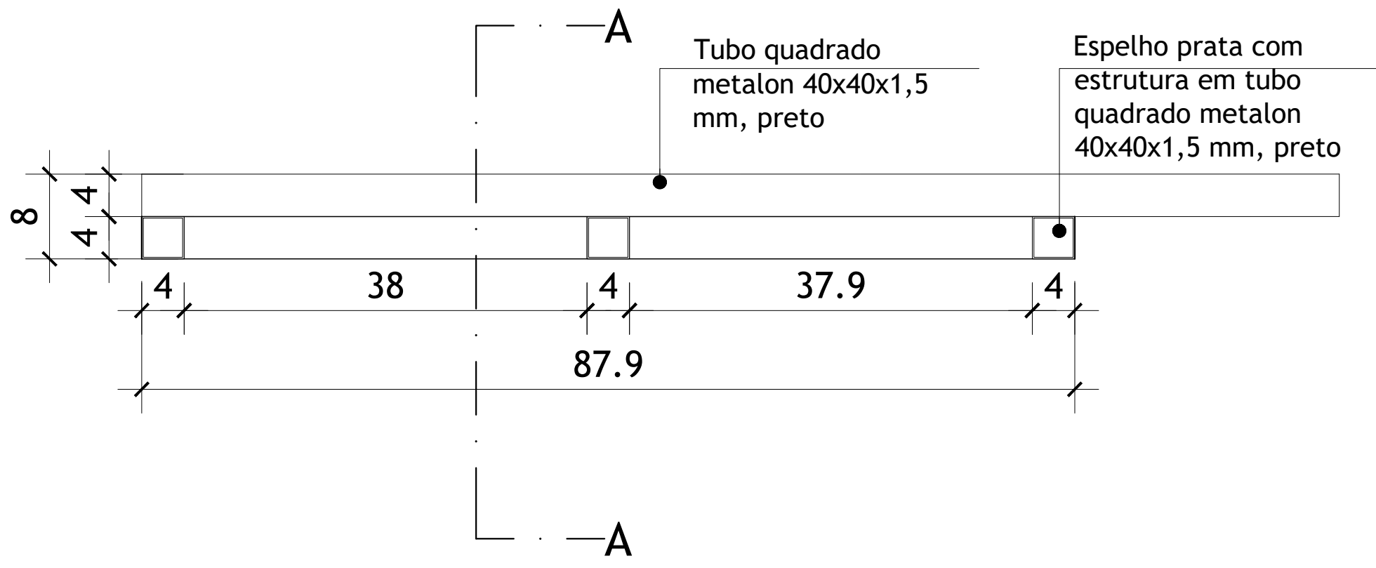
PLANTA ESPELHO ESCALA 1:5
