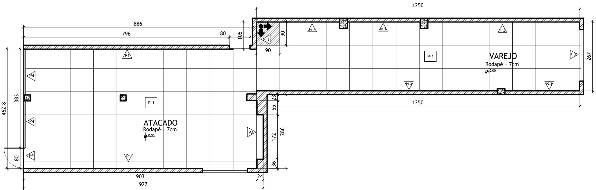
PLANTA DE ACABAMENTOS ESCALA: 1/75
