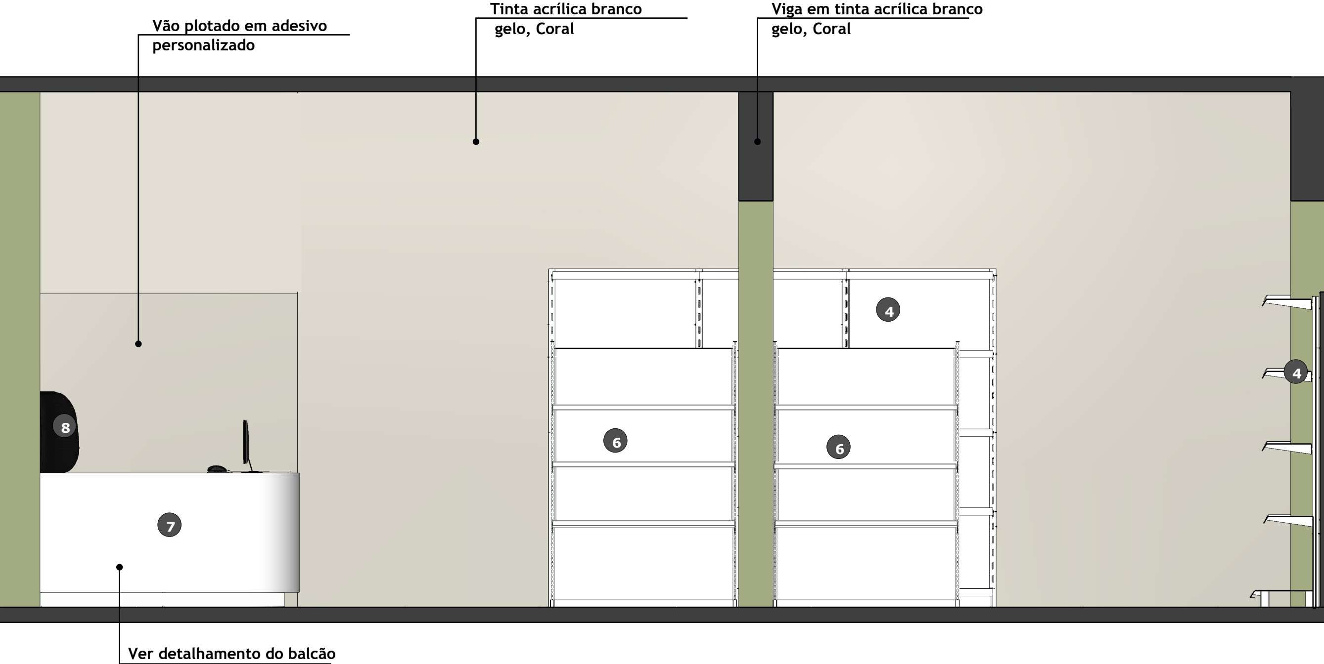
VISTA 6A - ESPECIFICAÇÕES ESCALA.: 1/25
