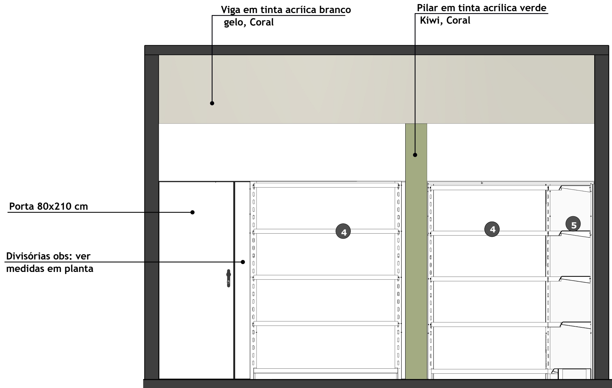
VISTA 5 - ESPECIFICAÇÕES ESCALA.: 1/25
