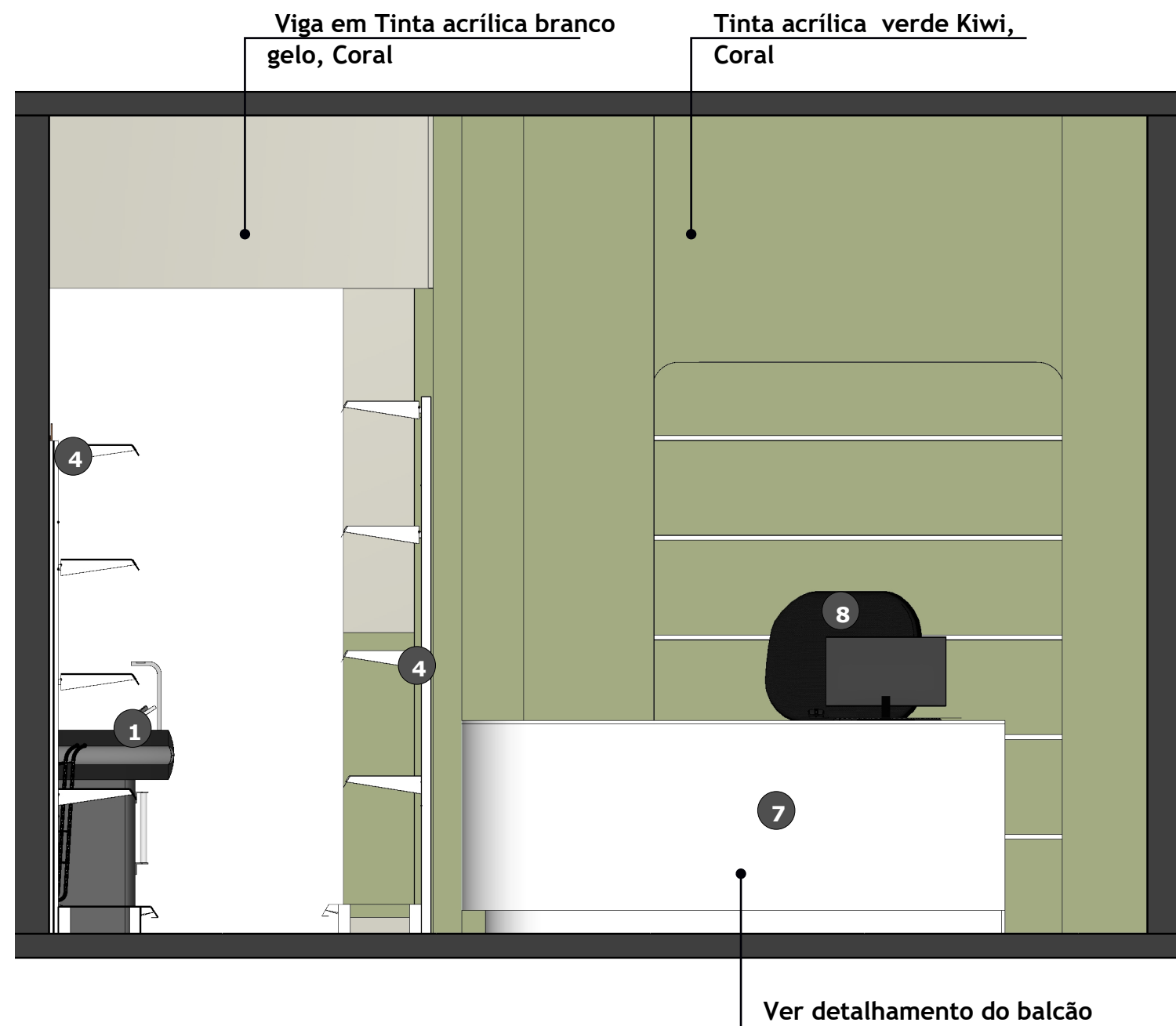
VISTA 7 - ESPECIFICAÇÕES ESCALA.: 1/25
